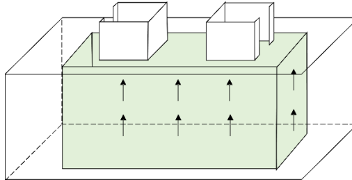
(d) Mode 3-Shearing of extrusion block
